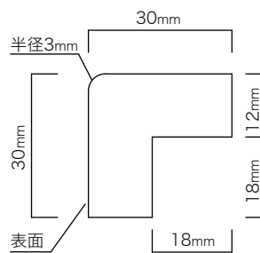
品 番 SY-36D サ イ ズ 30×30×3,650mm 出荷単位 1 ケース (4 本入) グレード 小節以上・人工乾燥 仕 上 り ブレーナー・無塗装
