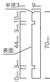
品番 SY-36H サイズ 9×70×3,650mm 出荷単位 1 ケース (4 枚入) グレード 小節以上・人工乾燥 仕上り プレーナー・無塗装
