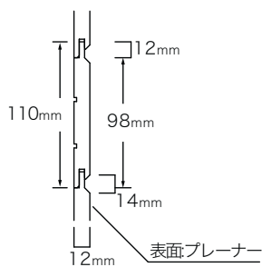
品番 SH-36STN サイズ 12×98mm（厚×有効巾） 長さ・㎡/枚 3,650mm(0.358㎡) 出荷単位 1 ケース (10 枚入) グレード 節有・人工乾燥 形状 メスカシ・本実 仕上り プレーナー・無塗装
