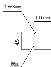
品番 SY-36I サイズ 14.5×14.5×3,650mm 出荷単位 1 ケース (4 本入) グレード 小節以上・人工乾燥 仕上り プレーナー・無塗装
