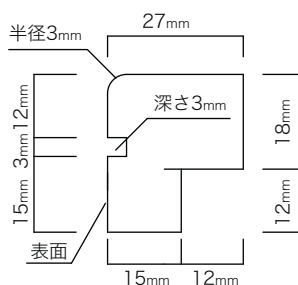
品 番 SY-36M サ イ ズ 27×30×3,650mm 出荷単位 1 ケース (4 本入) グレード 小節以上・人工乾燥 仕 上 り プレーナー・無塗装
