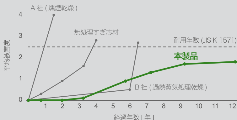
野外杭試験による耐用年数の評価(ハルキ編集)
