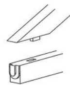
下端部合噛ほぞ差し
